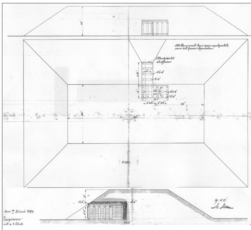
Jordvolden med det indbyggede ammunitionsdepot. Øverst i længdesnit, i midten set ovenfra og nederst i tværsnit. Målene er angivet i fod og tommer (hvh. ' og '')
