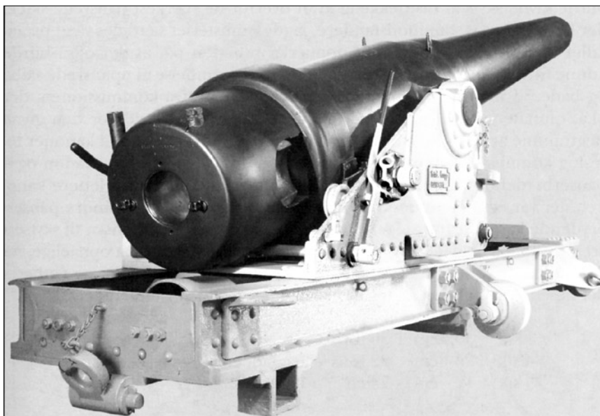
Den 6" 80 ctr. bagladekanon. Foto: Helge Abrahamson, TM
