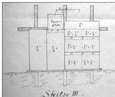
Galgen med de forskellige stålplader
