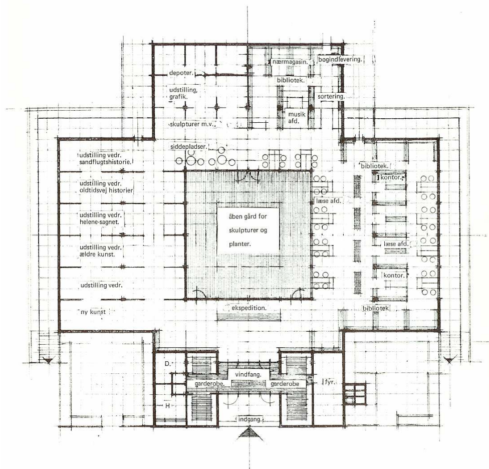
Stueplan i det foreslåede kulturhus.
