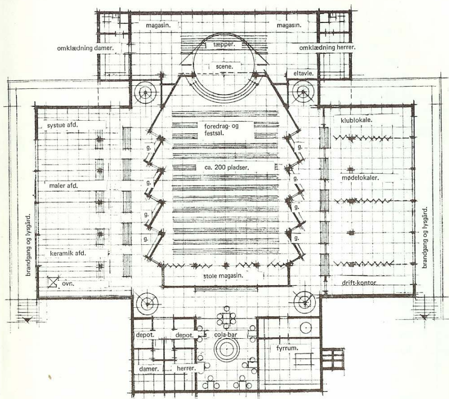
Kælderplan i det foreslåede kulturhus.
